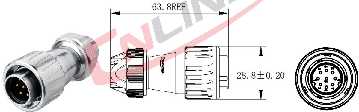
DZ-20-CXXPE-03-001A DZ20 系列公插头焊接式金属款
